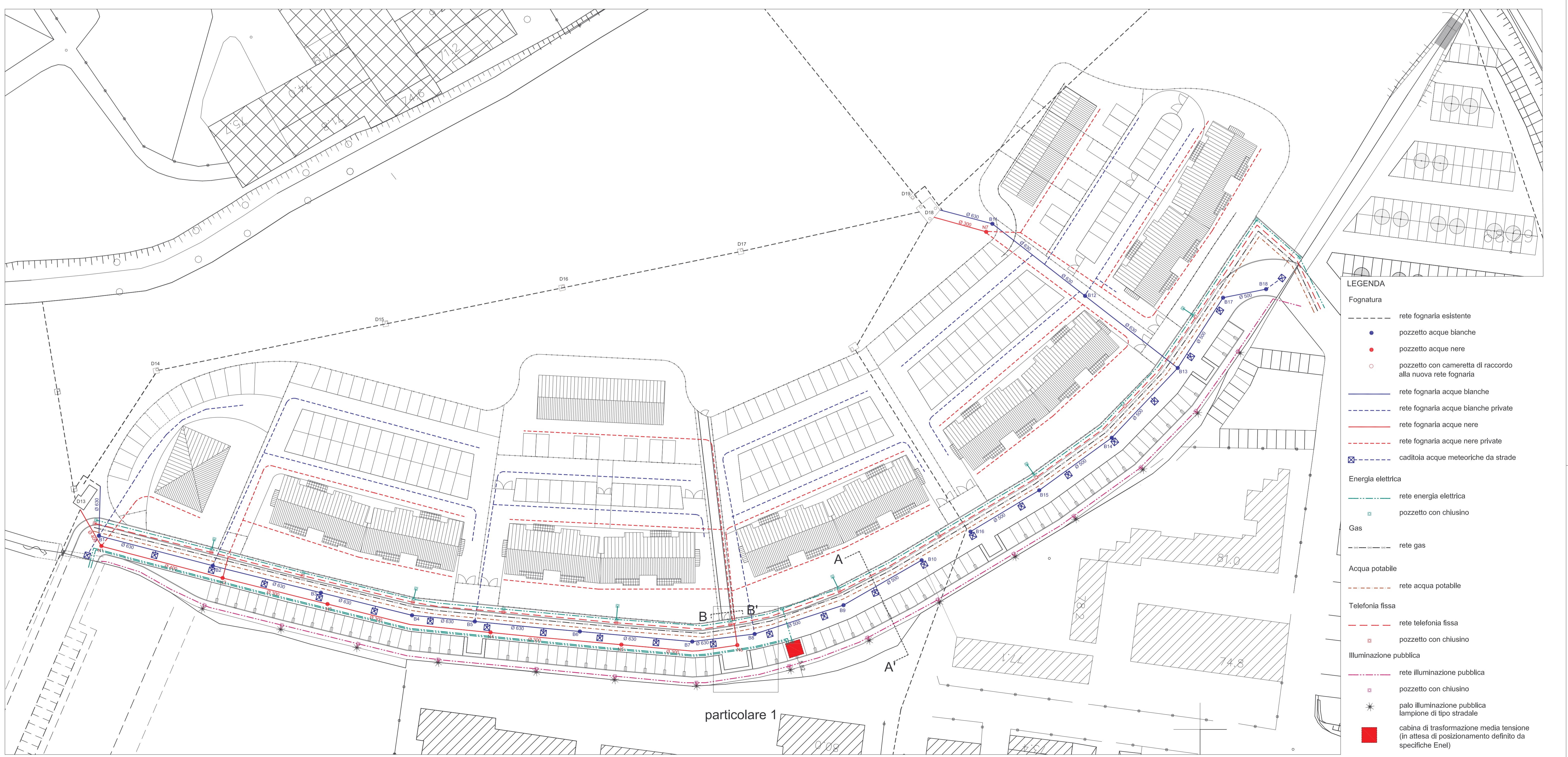
schema reti interrate - scala 1:500
