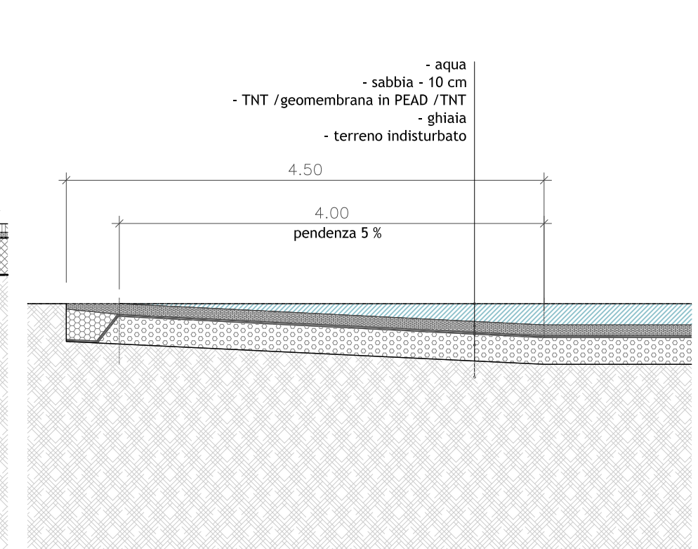
D3. Dettaglio 1 -Stagno 1:50
