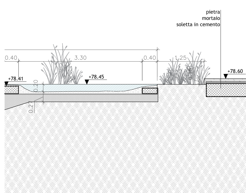
D2. Dettaglio 2 -Stagno 1:50
