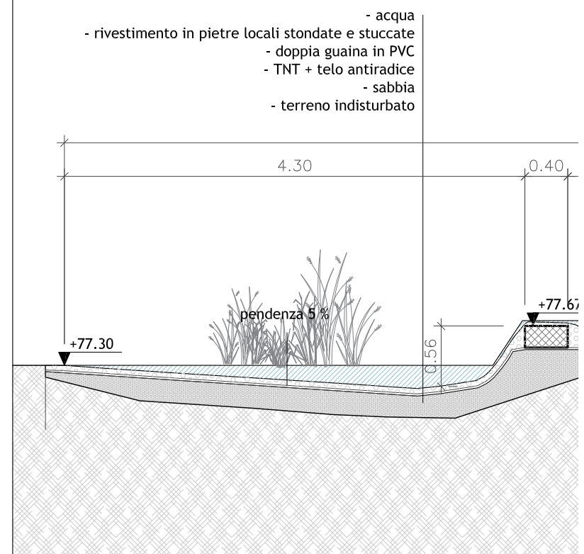
D1. Dettaglio 1 -Stagno 1:50
