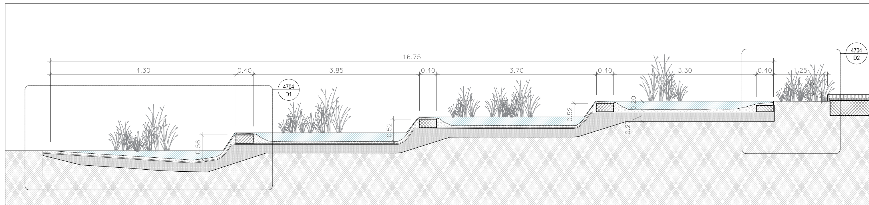
1. Sezione AA Stagno 1:50
