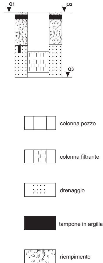
Schema pozzo progetto
