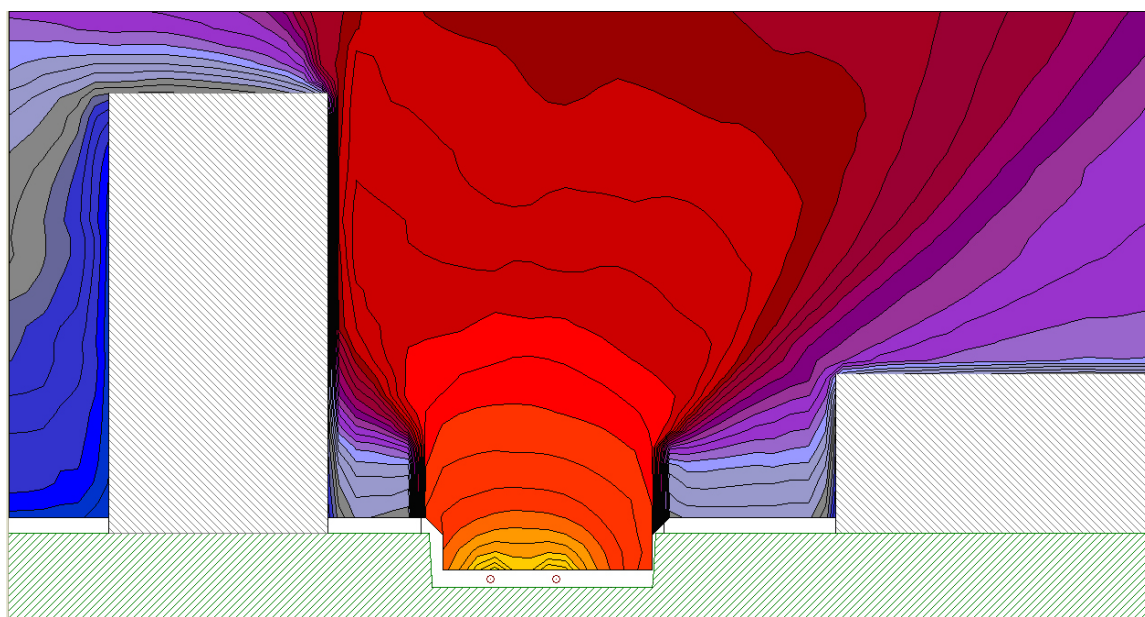
Stato di progetto – Sezione 4
