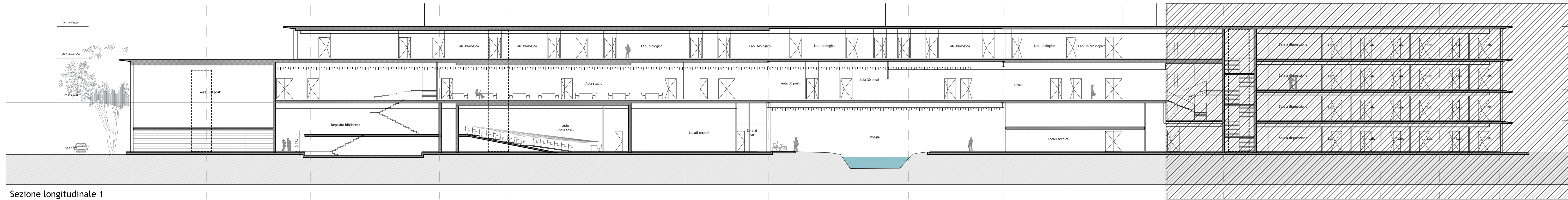
Sezione longitudinale 1
