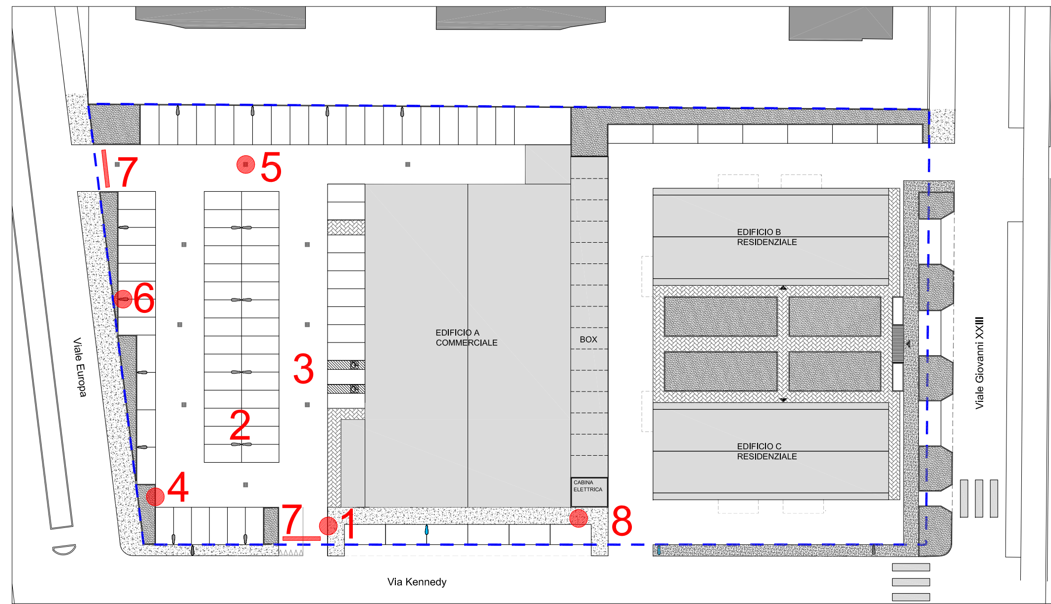
PIANTA CHIAVE Scala 1:500
