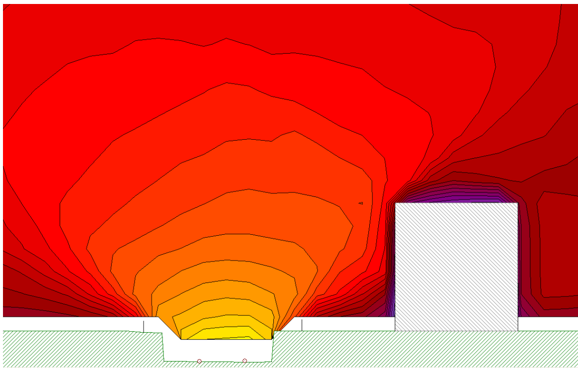
Stato di fatto – Sezione 2
