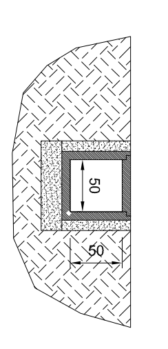
Cunicolo Tubazione Melano
