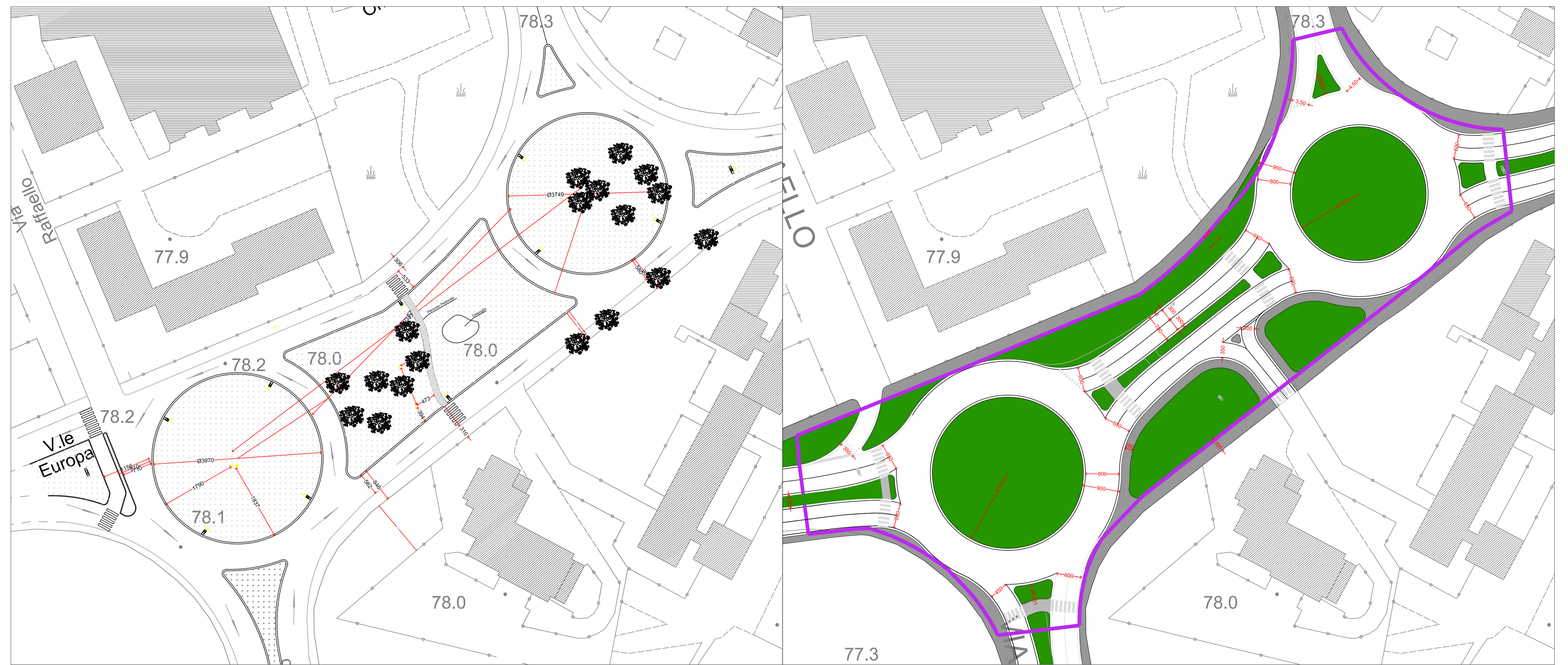
E - NUOVA INTERSEZIONE A ROTATORIA - STATO DI FATTO
