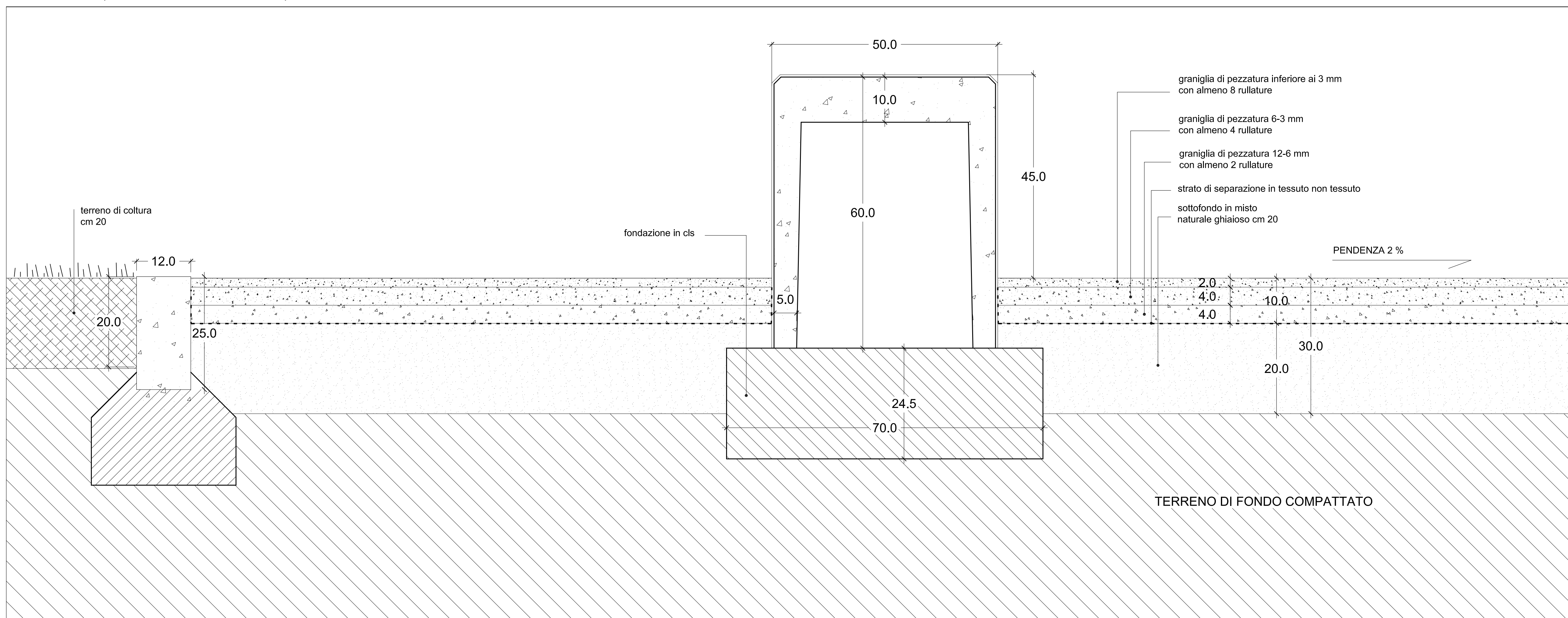
Particolare 2 (elemento di seduta in cls) scala 1 : 5
