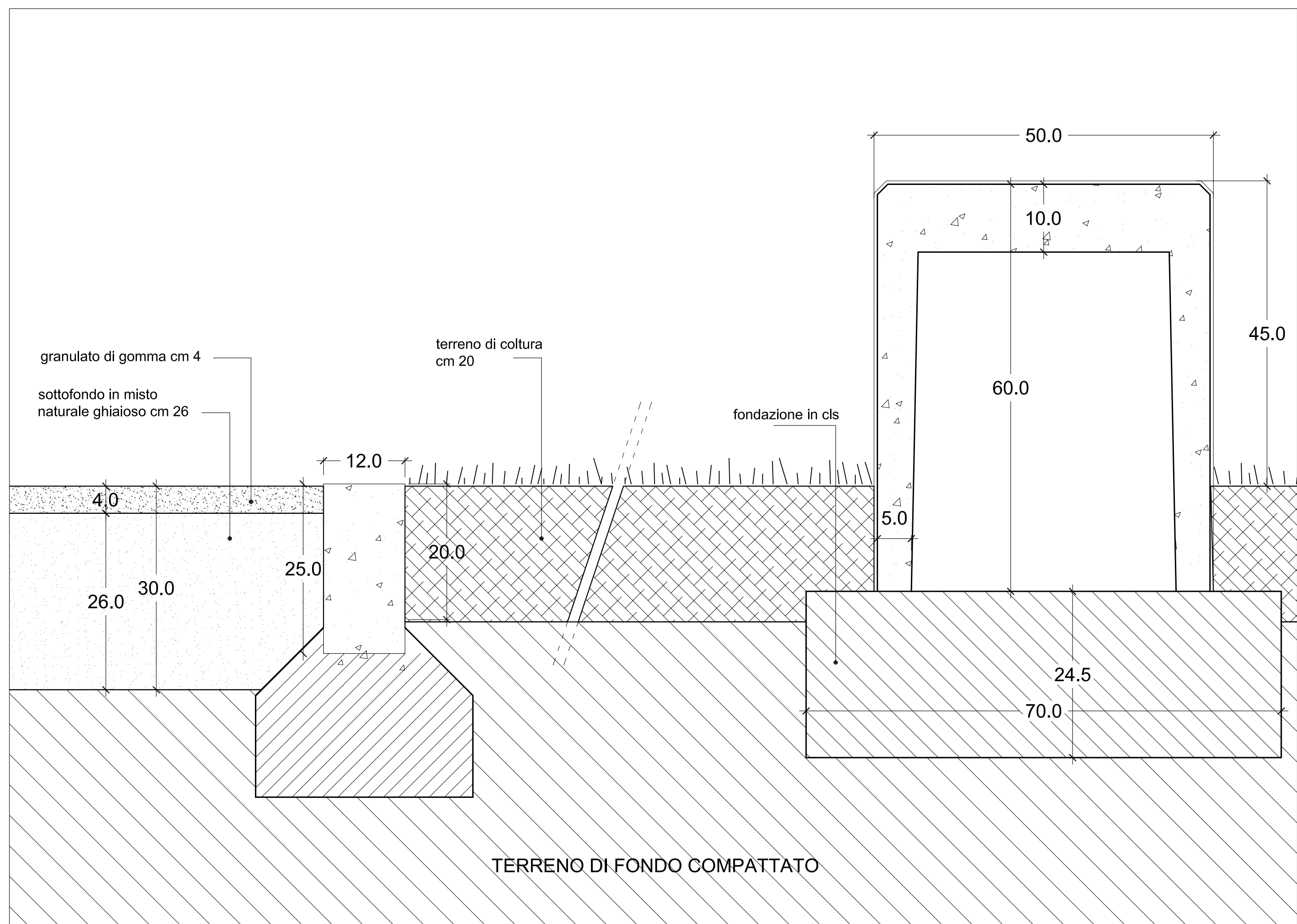
Particolare 1 (pavimentazione antitrauma) scala 1 : 5
