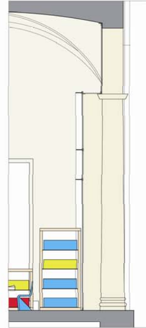
Dettaglio Vetrata s. 1:20
