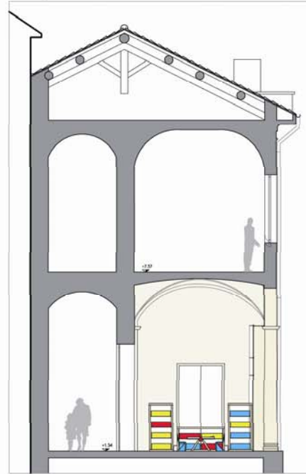
Sezione B,B s. 1:50
