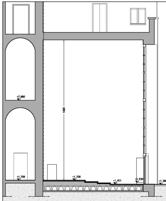
Sezione B_B
