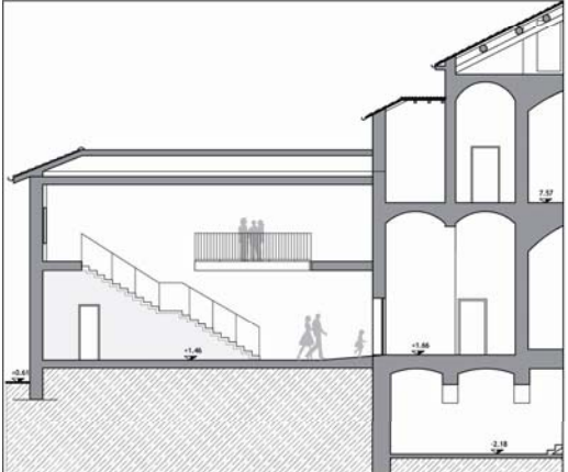
Sezione C1_C1
