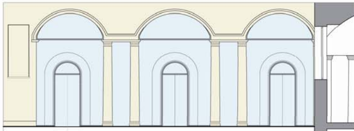
Vista esterna s. 1:50
