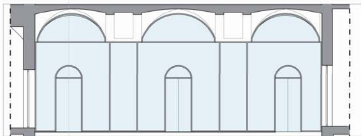
Vista interna s. 1:50
