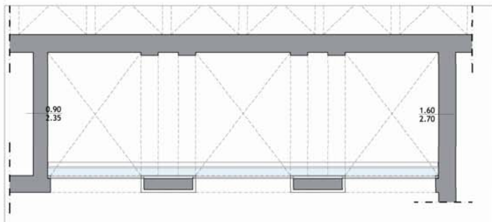
Sezione D,D s. 1:50
