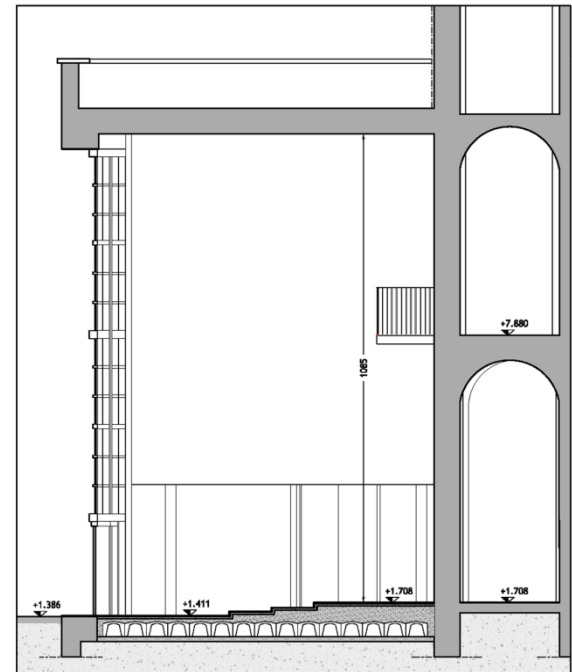
Sezione B1_B1
