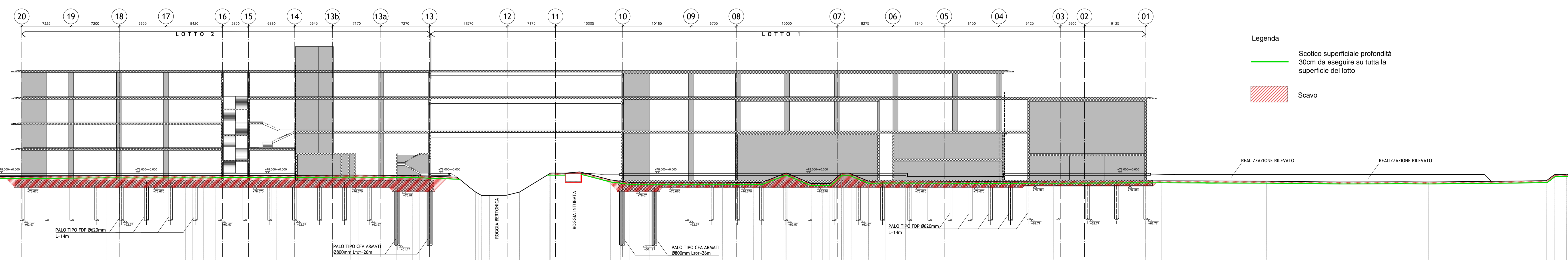
SEZIONE 2-2 Scala 1:250
